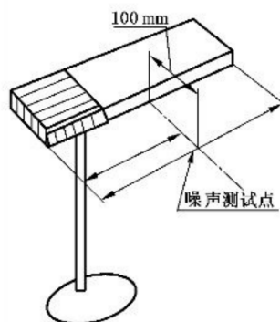
图 5 灯罩噪声测试点
