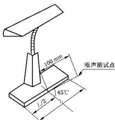
图 4 底座噪声测试点
