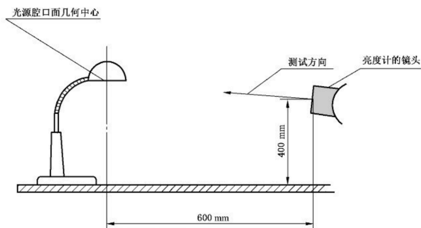
图1 遮光性试验观察方式的侧视图
